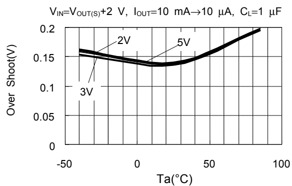
负载变动过冲的温度依存性
