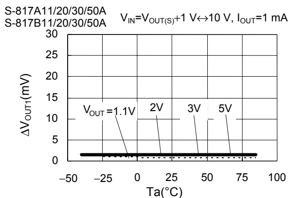
(6) 输入稳定度1—周围温度
