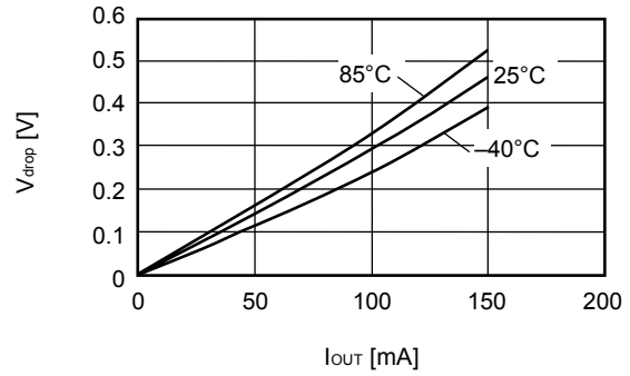
S-1323B30
